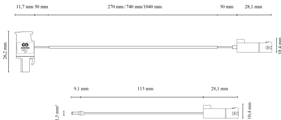
Struktur- und Maßdarstellung der Kabelkonfektion. Maße gemäß Quellzeichnung.
